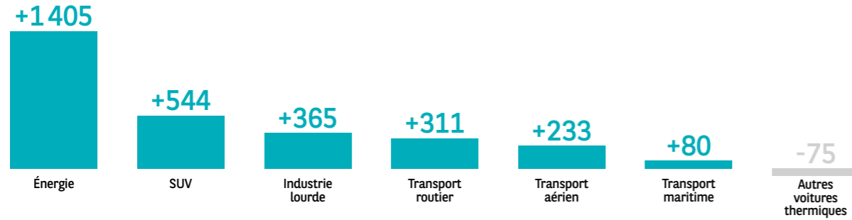
ÉVOLUTION DES ÉMISSIONS (MT CO 2 )
